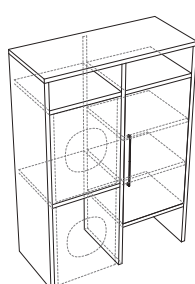
145,6x65x h210 cm colonna con ante porta lavatrice+asciugatrice + ripiani column for washing machine + dryer + shelves
