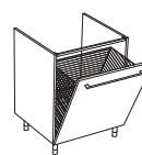
67,1x63x h87,2 cm modulo con cesto portabiancheria module with laundry basket
