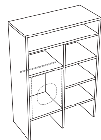
145,6x65x h210 cm colonna portalavatrice/ asciugatrice + ripiani washer / dryer door column + shelves
