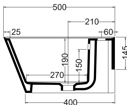
SEZIONE A-A'
