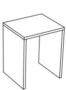
75x65x h91 cm struttura a giorno per inserimento modulo open structure for 1 module
