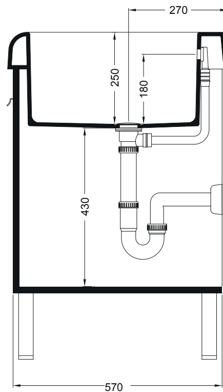
SEZIONE A-A
