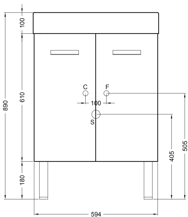
VISTA FRONTALE
