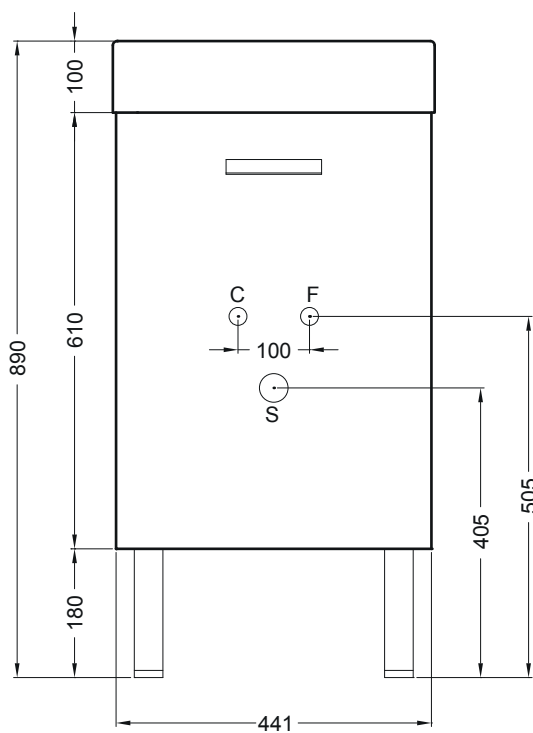
VISTA FRONTALE
