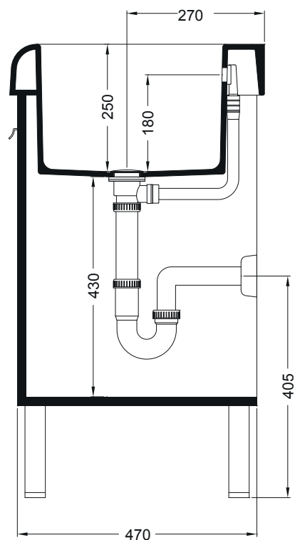
SEZIONE A-A
