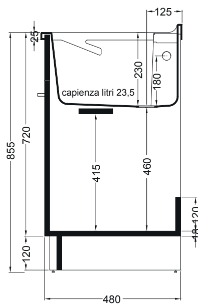
SEZIONE A-A'
