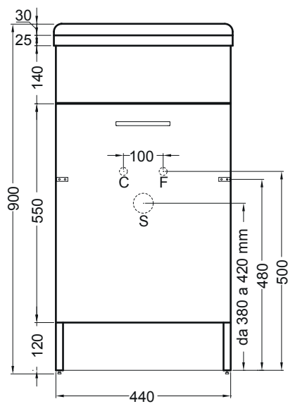
VISTA FRONTALE
