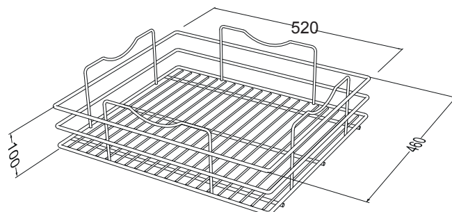
CESTO ESTRAIBILE
