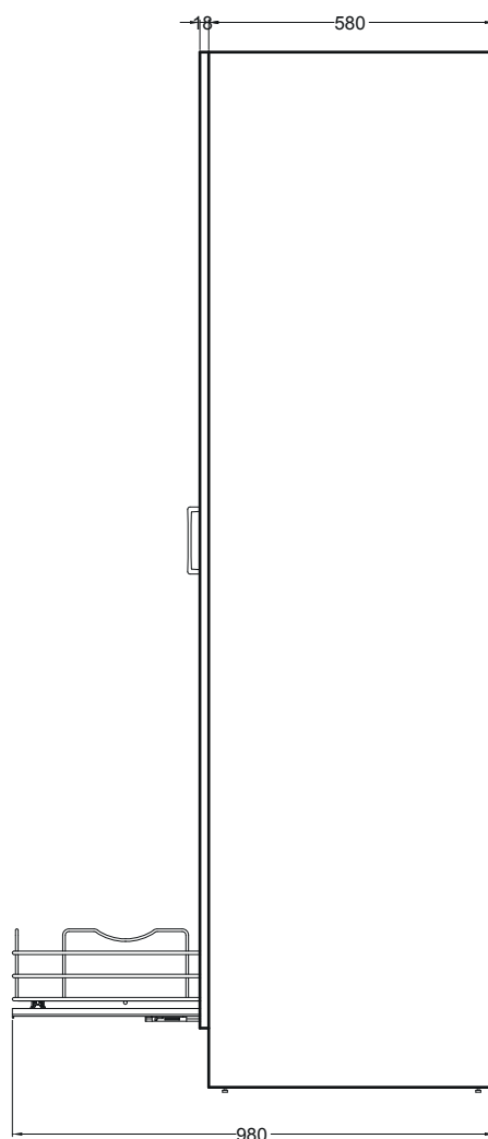
VISTA LATERALE
