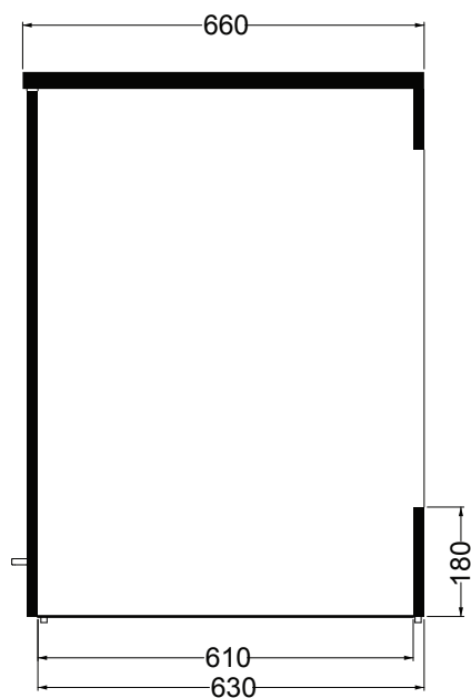
SEZIONE A-A'
