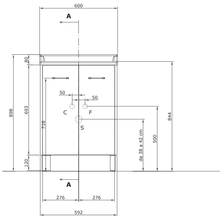
VISTA FRONTALE
