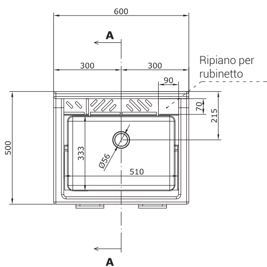
PIANTA
