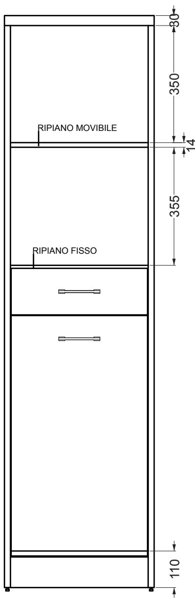
VISTA FRONTALE SENZA ANTE
