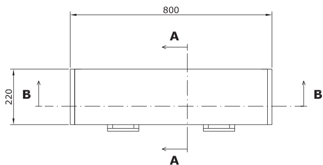
PIANTA
