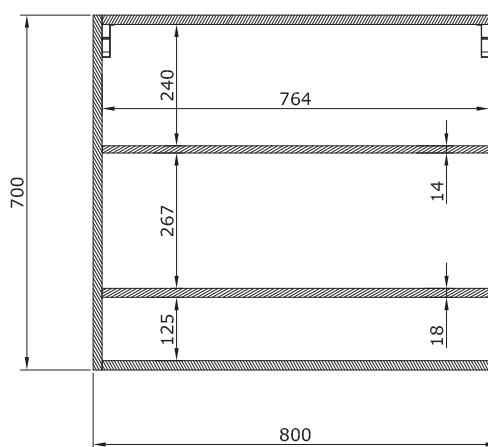
SEZIONE B-B
