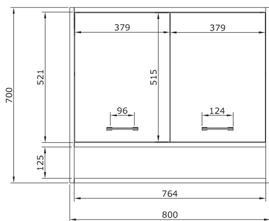
VISTA FRONTALE
