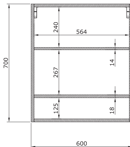
SEZIONE B-B
