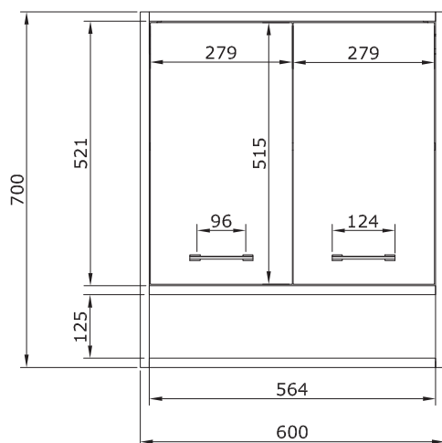
VISTA FRONTALE
