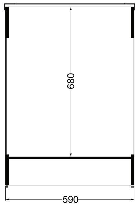
SEZIONE A-A
