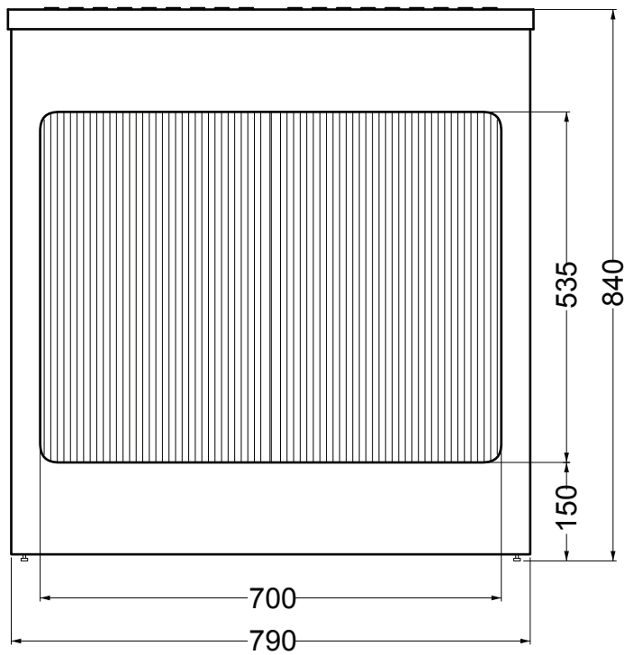
VISTA FRONTALE
