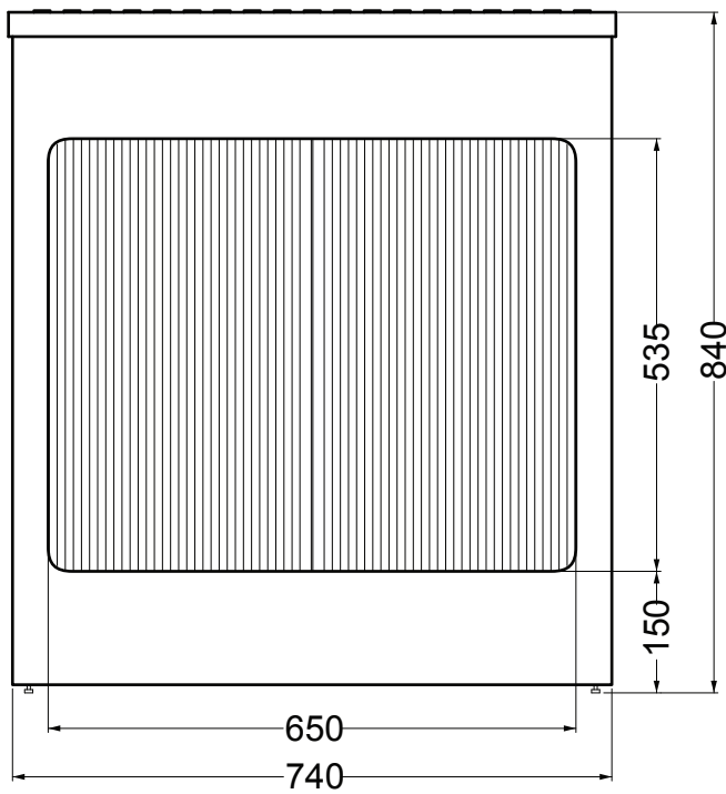
VISTA FRONTALE
