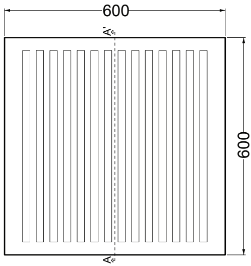
PIANTA
