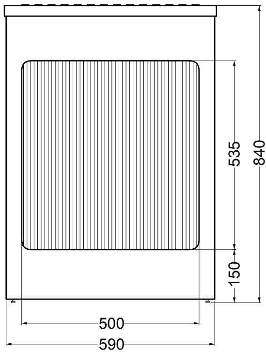
VISTA FRONTALE
