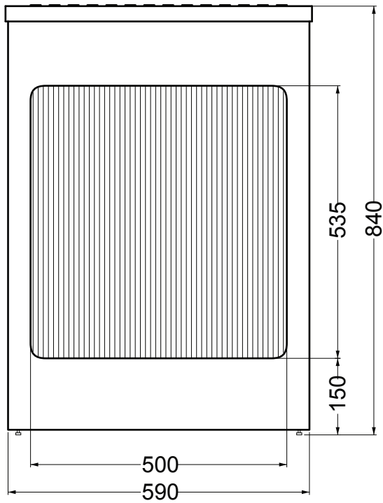
VISTA FRONTALE
