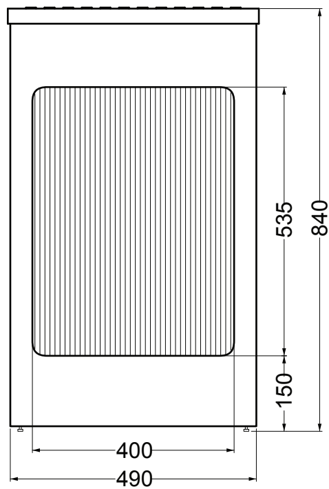
VISTA FRONTALE
