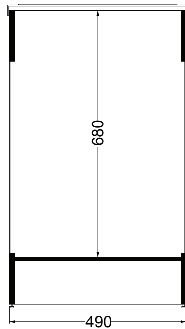
SEZIONE A-A
