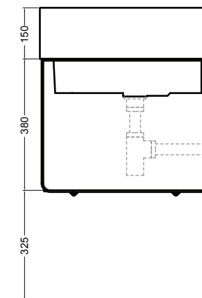
VISTA LATERALE
