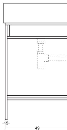
SEZIONE B-B
