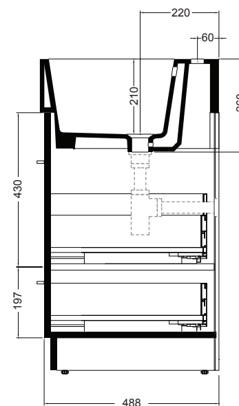
SEZIONE B-B
