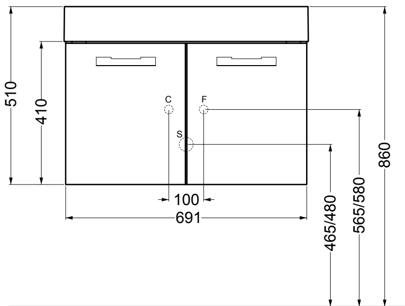
VISTA FRONTALE
