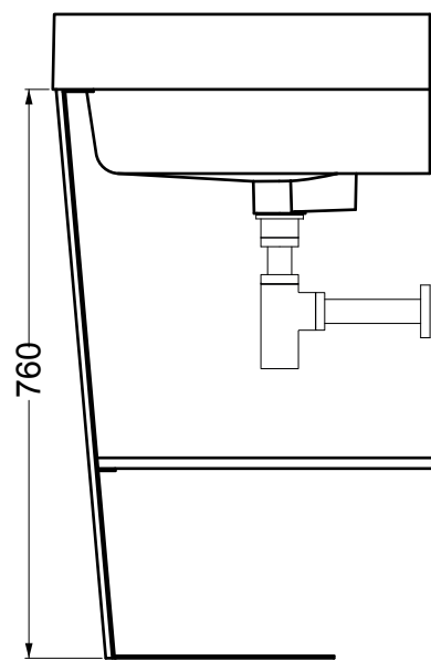
VISTA LATERALE
