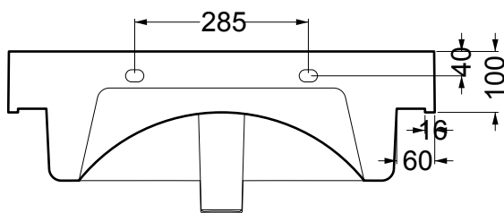
VISTA POSTERIORE
