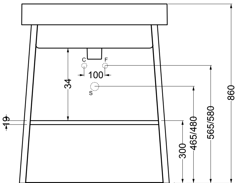
VISTA FRONTALE
