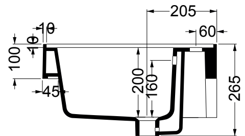
SEZIONE A-A'
