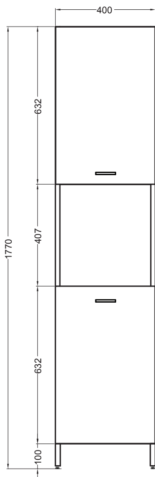
VISTA FRONTALE
