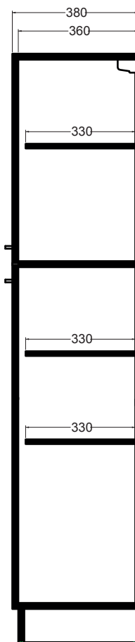
SEZIONE A-A
