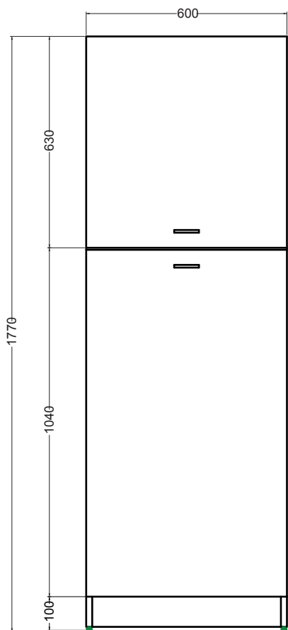
VISTA FRONTALE
